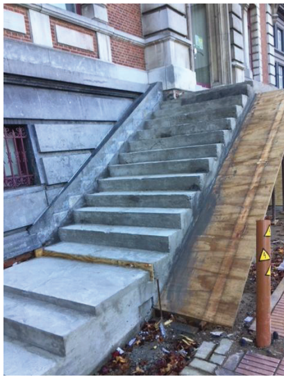
De betonconstructie van de nieuwe pui.
